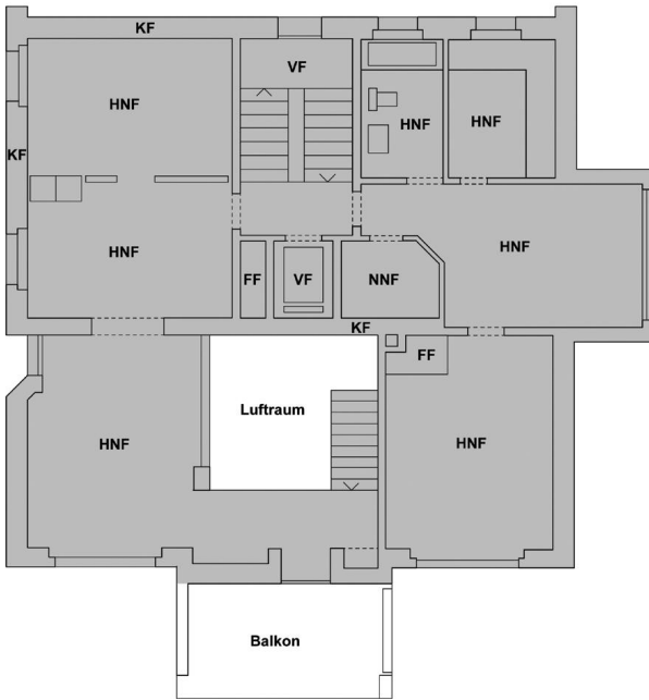
Grundriss 1. Obergeschoss:
