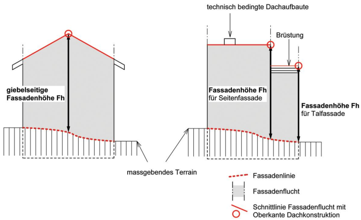
Figur 5.2 Fassadenhöhe
