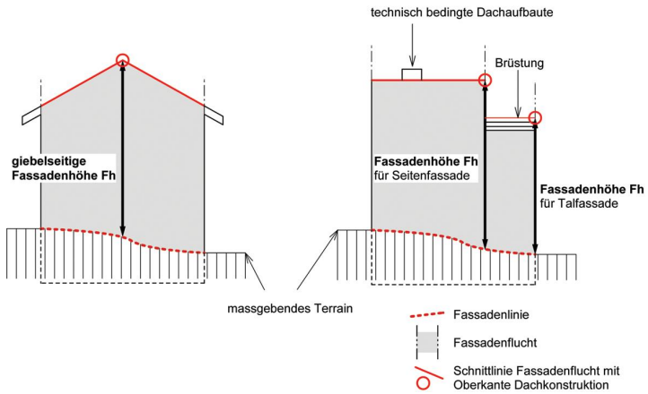
Figur 5.2 Fassadenhöhe
