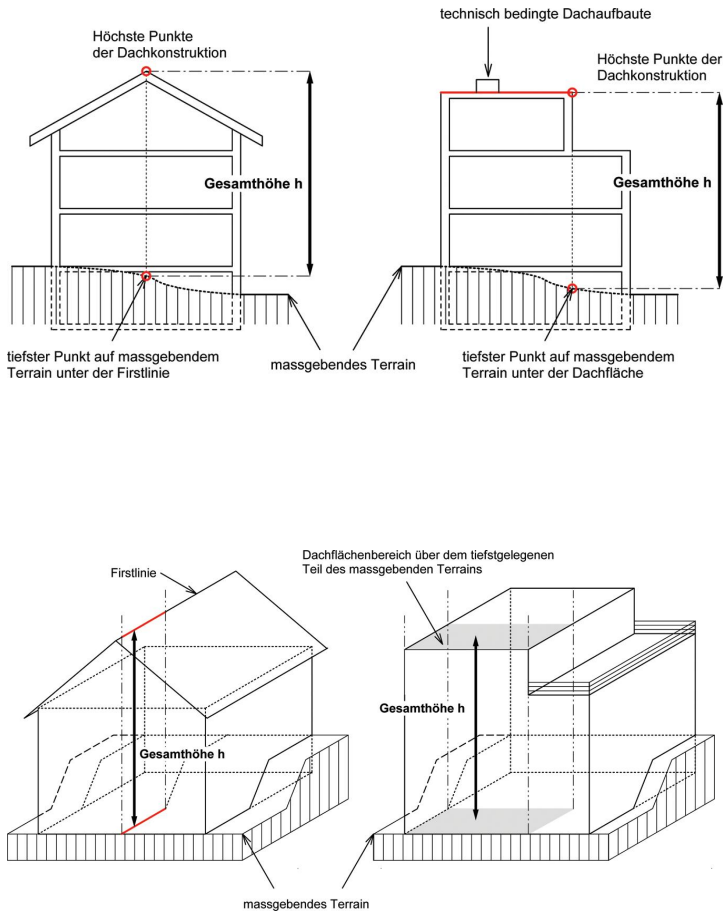
Figur 5.1 Gesamthöhe
