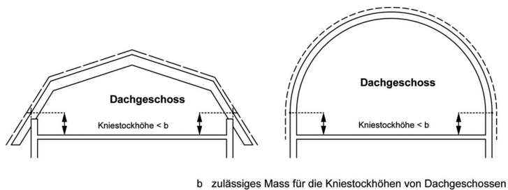
Figur 6.3 Dachgeschosse
