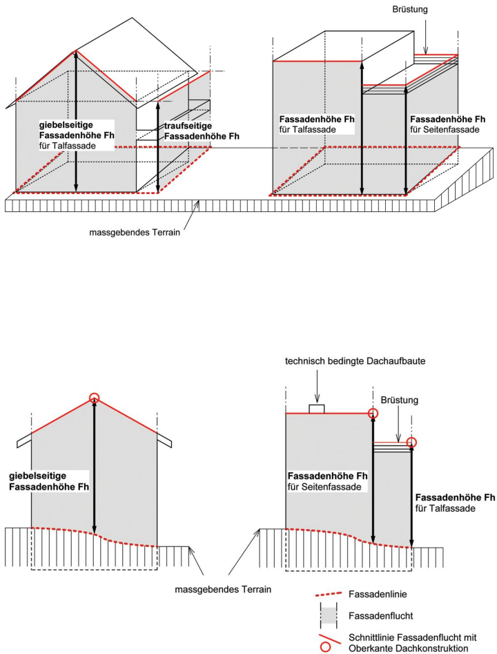
Figur 5.2 Fassadenhöhe
