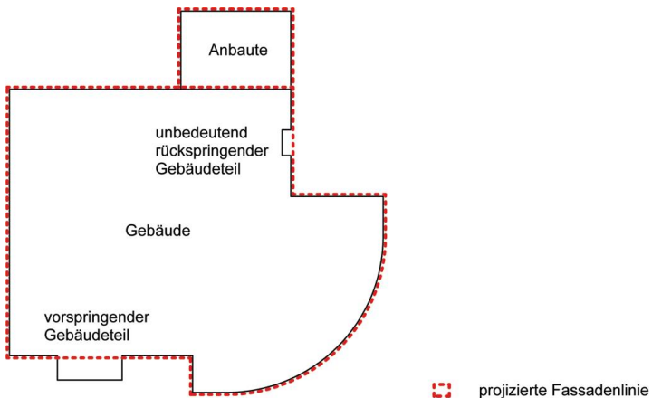
Figur 3.3 Projizierte Fassadenlinie
