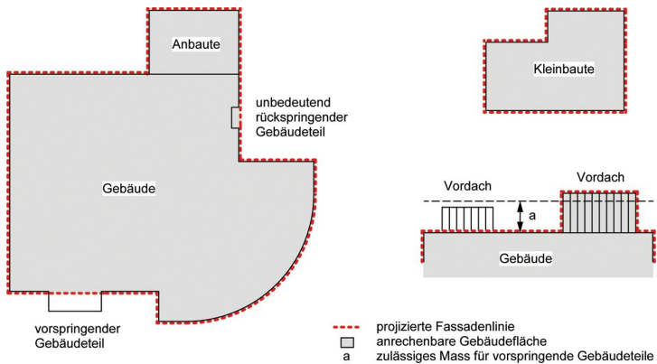
Figur 8.4 Anrechenbare Gebäudefläche
