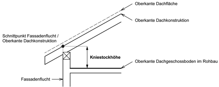
Figur 5.3 Kniestockhöhe
