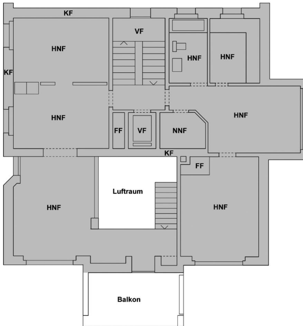
Grundriss 1. Obergeschoss:
